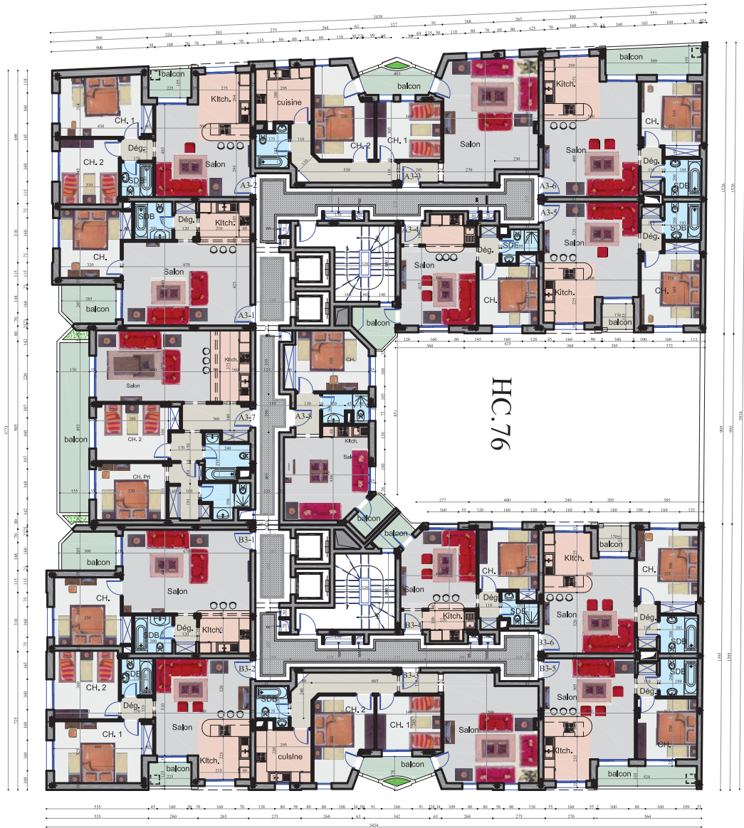
Plan 3ème étage
